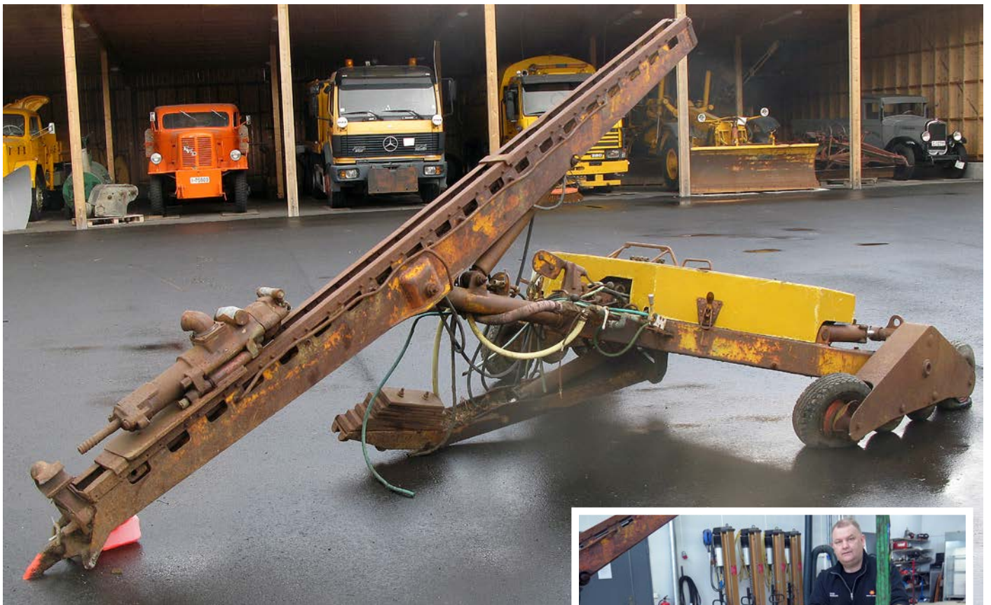
Geita fra 1974 før oppussing ved vegmuseet. Den ble sist brukt ved byggingen av Atlanterhavsvegen i 1988. Foto: Mass Haugen, Norsk vegmuseum.
